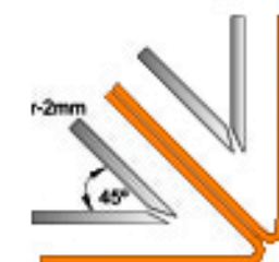
Ranura de 90° ( forma de V ) de doblez hasta 90°
