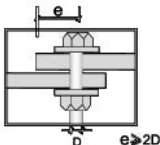
Atornillado
