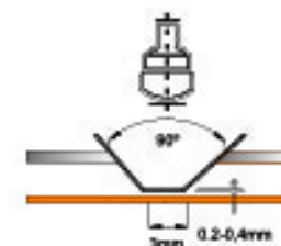
Ranura de 90° ( forma de V ) de doblez hasta 90°
