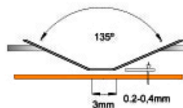
Rauter común con broca apropiada
