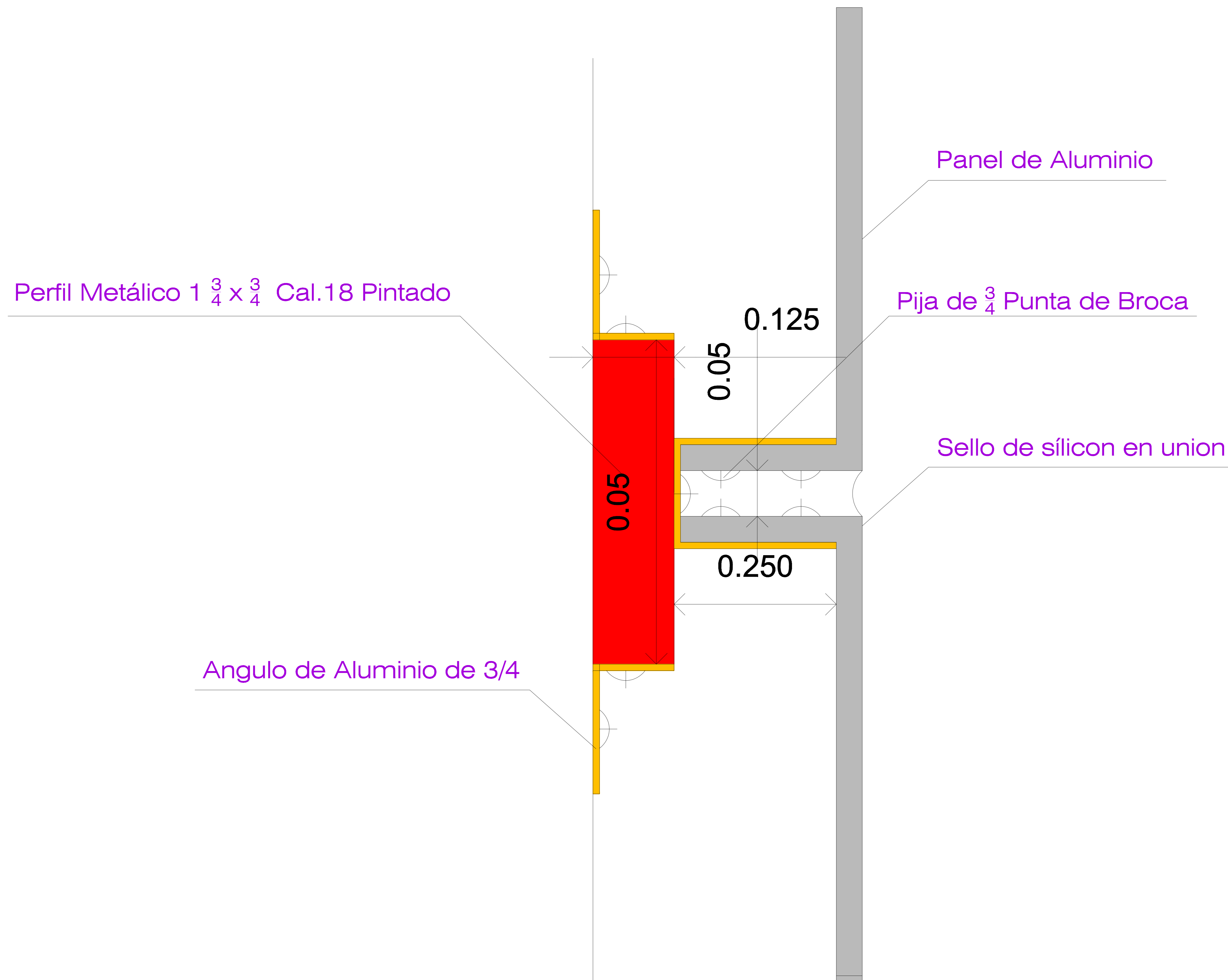
Detalle A-1
