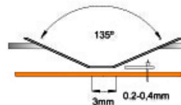
Rauter común con broca apropiada
