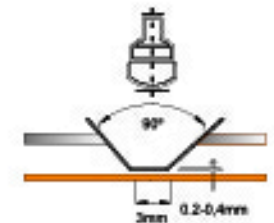
Ranura de 90° ( forma de V ) de doblez hasta 90°
