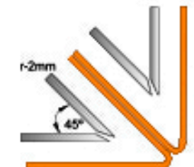
No es adecuado para ICOBOND ranurar rectangularmente, por dobleces de hasta 150° depende del espesor del panel.
