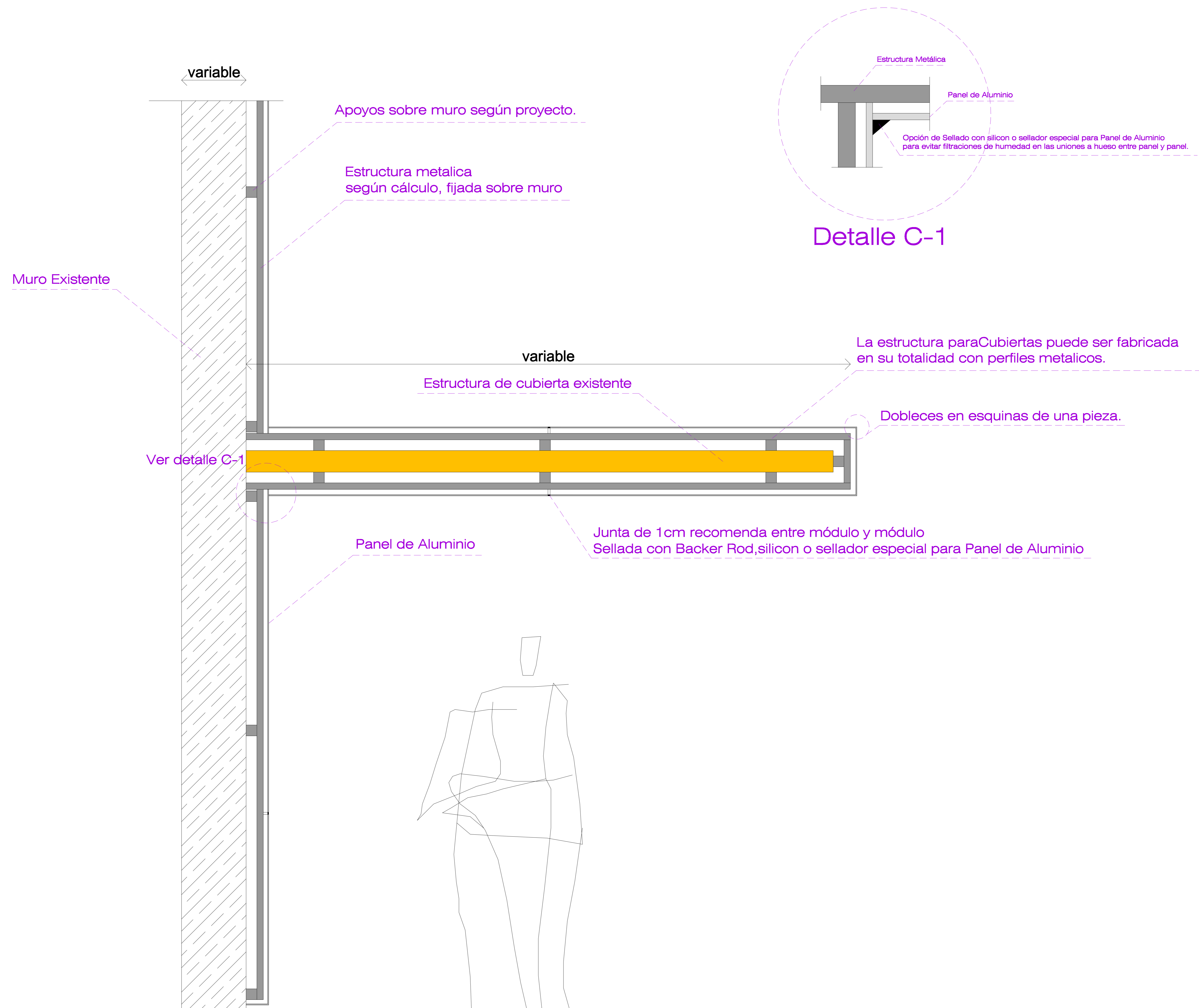
Corte Lateral Tipo.
